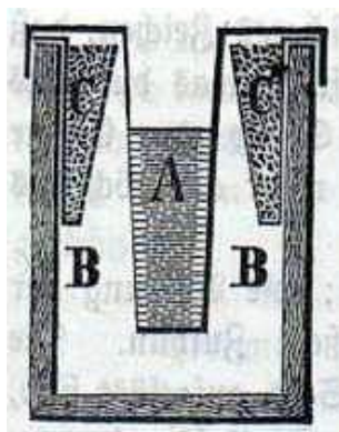
Original Schemazeichnung der Eisbüchse Meidinger: A Friergefäß, B Kühlgefäß, C Salzbehälter
